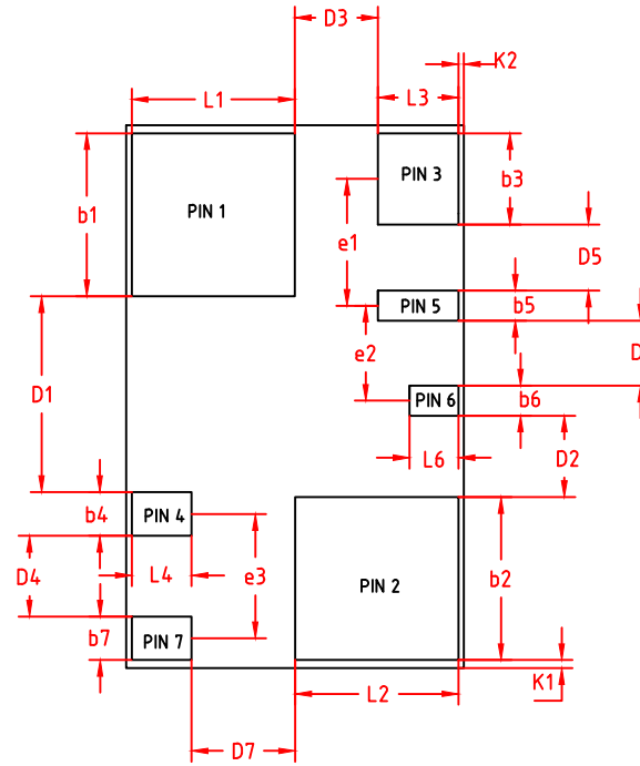
BOTTOM VIEW 背视图
