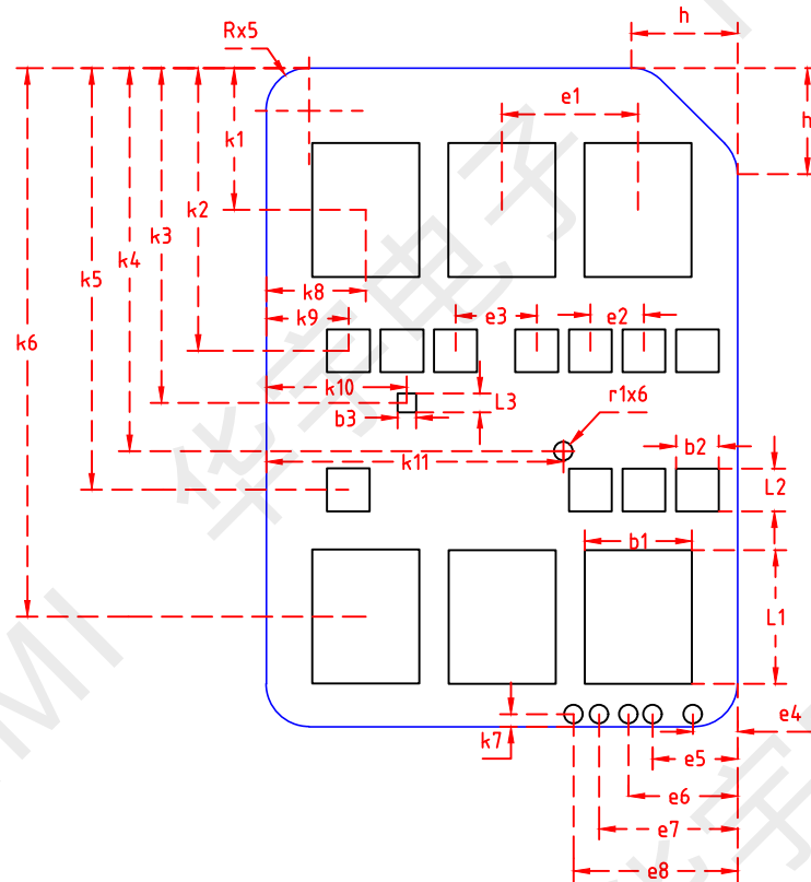
BOTTOM VIEW 背视图
